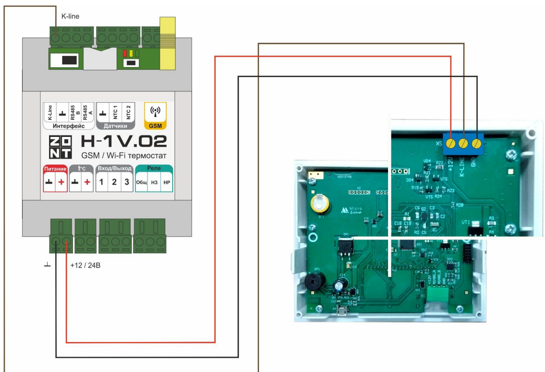
Интерфейс K-Line
